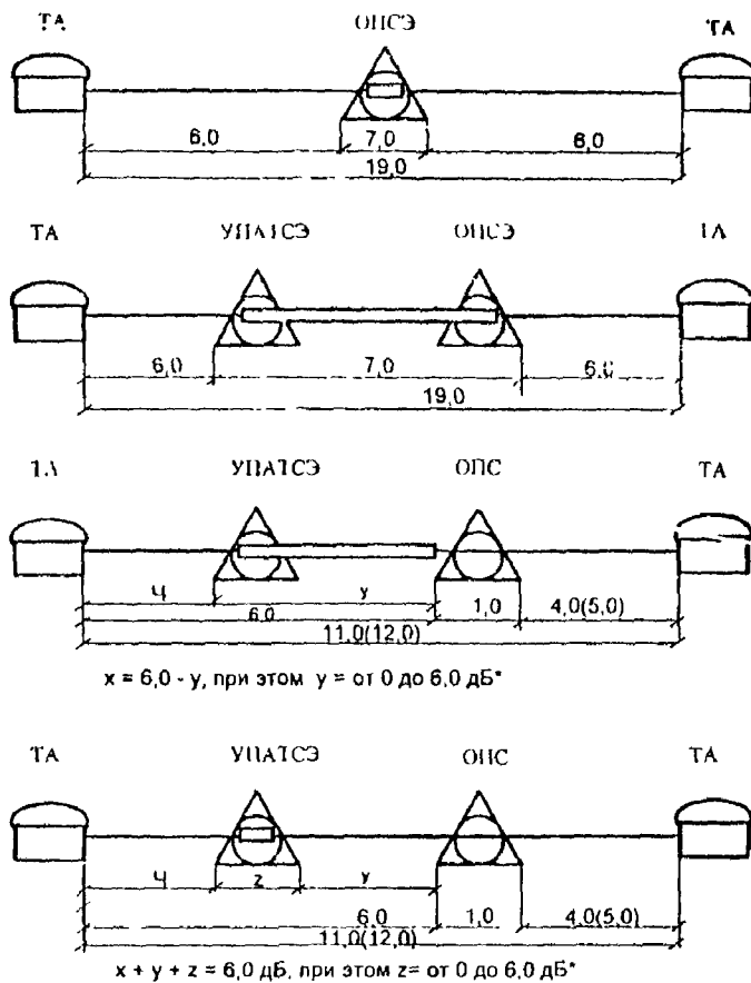
Рисунок Б.1 – Распределение норм затухания на перфорированной сегни, лист 1
