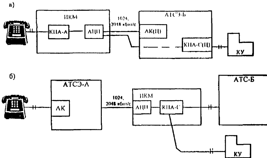
Рисунок 6.5 Реализация на АТСЭ-Б цифрового абонентского комплекта для подключения прямого абонента
