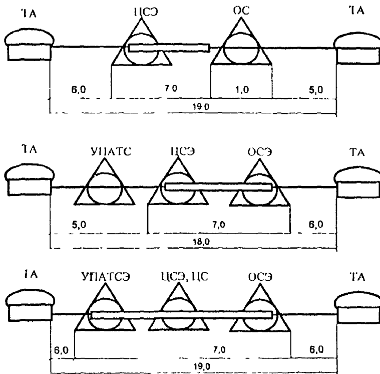
Рисунок Б 9 – Распределение норм затухания на СТС при одноступенчатом радиальном построении
