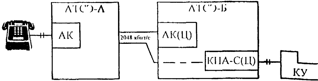
Рисунок 6.5 Реализация на АТСЭ-Б цифрового абонентского комплекта для подключения прямого абонента
